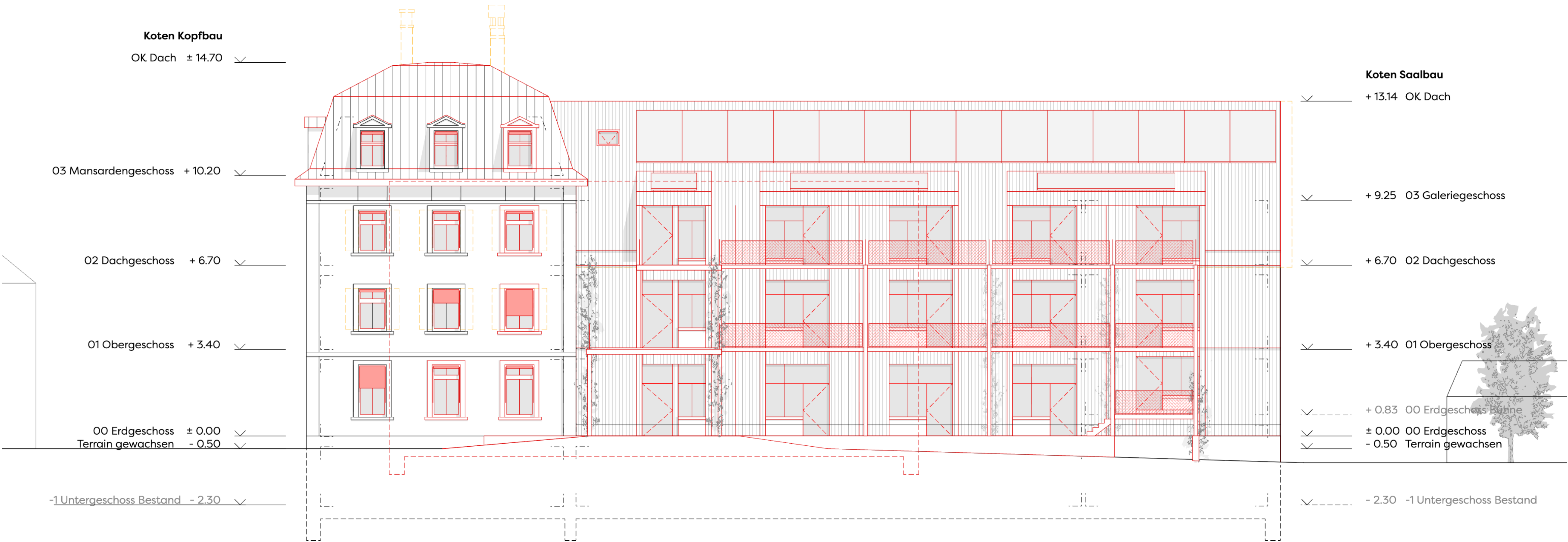
Ansicht Kopfbau und Saalbau
