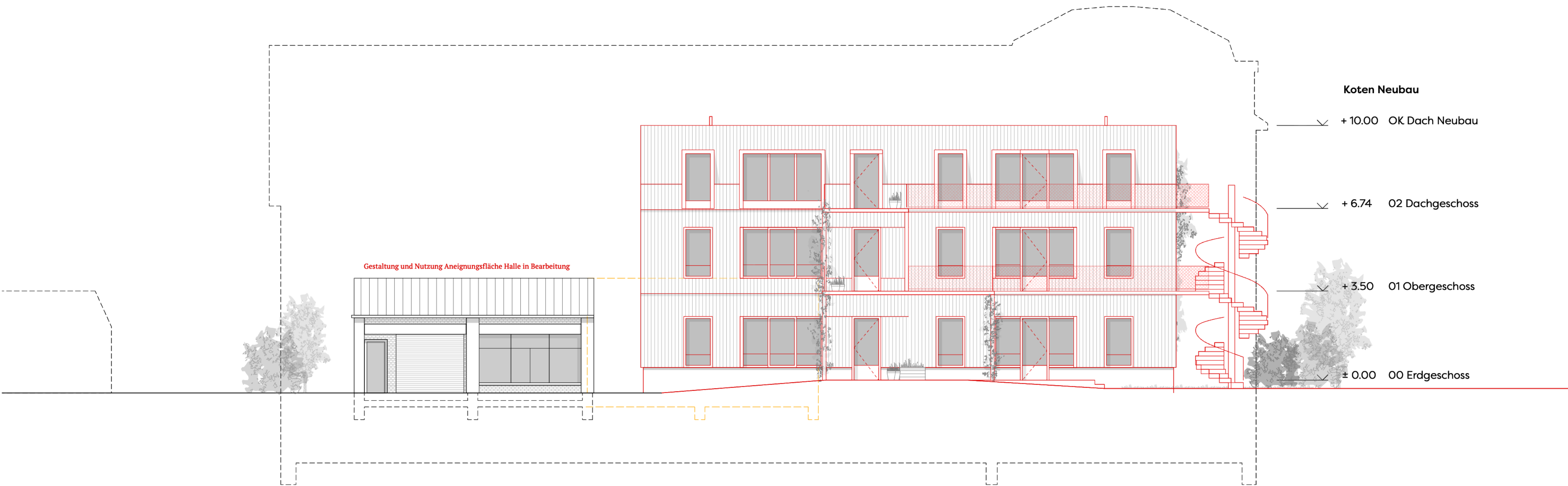
Ansicht Neubau
